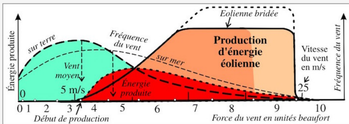
Schéma théorique de la courbe de puissance d'une éolienne selon la vitesse du vent.
