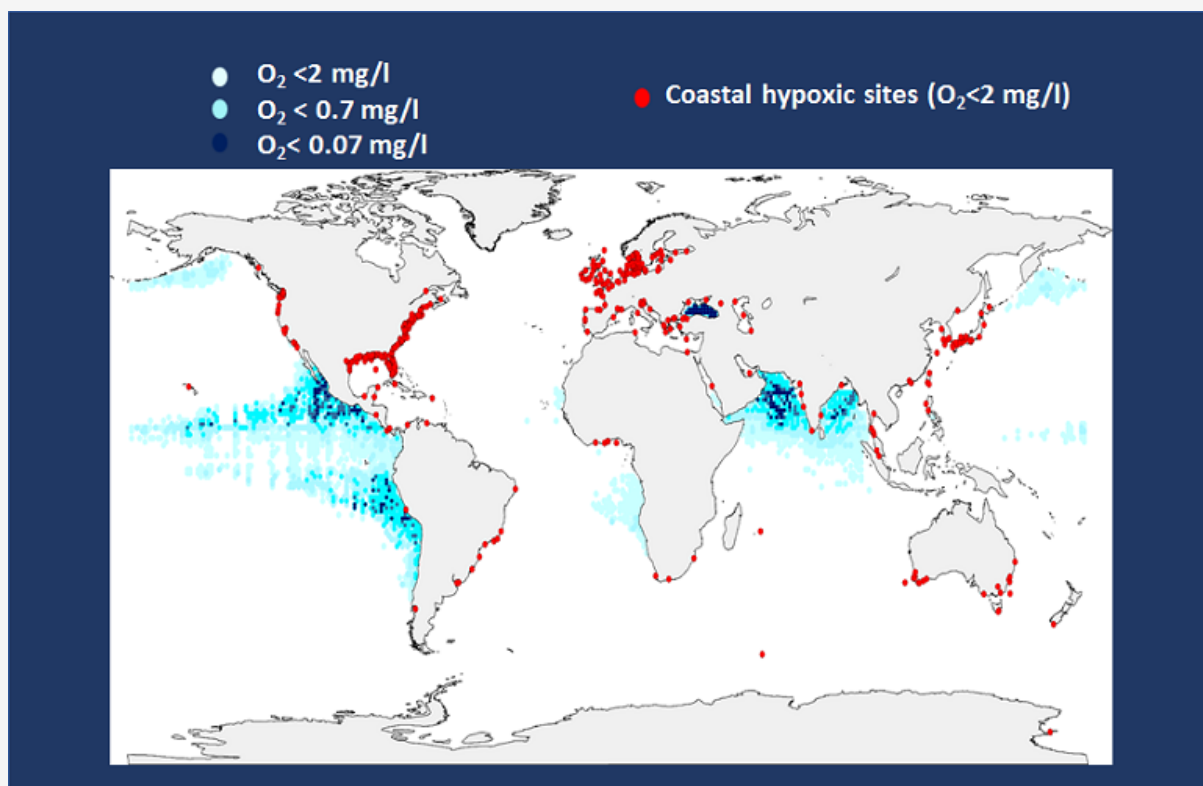
La carte des zones côtières hypoxiques, publiée dans Science.
